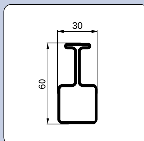
Váha 3,7 kg/m Weight 3,7 kg/m
