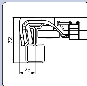
Pohled na příčník Shown with roof construction
