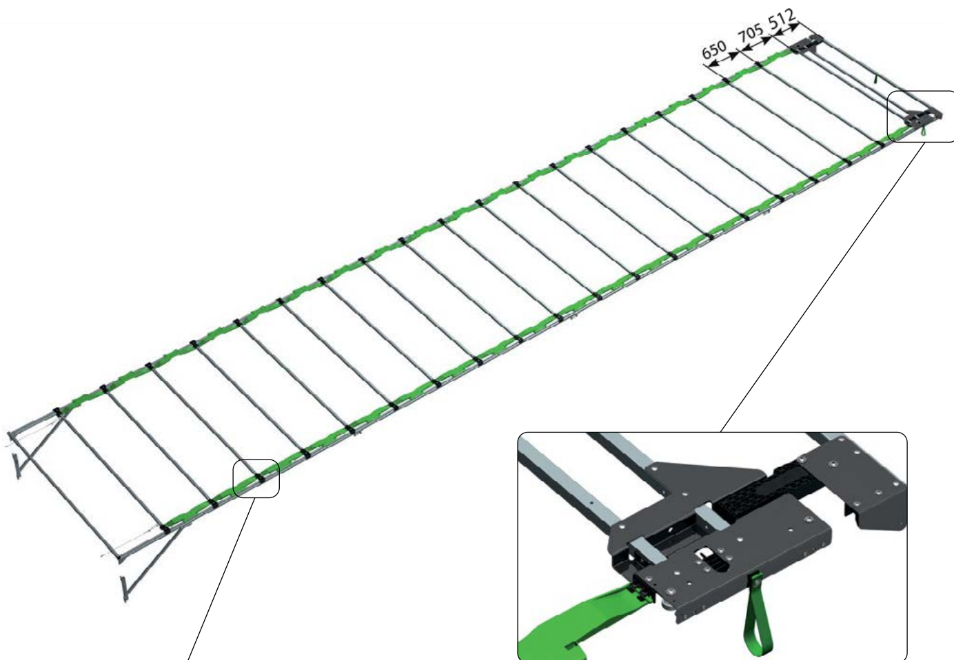
Koncový pojezd s automatickým zvedáním a zakončením End carriage with automatic fold up and end bow
