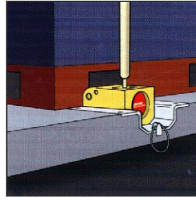
Jazdec je dole, náklad je položený na podlahe
