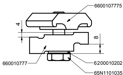
Obr. č. 1. 6600197778 Svorka hliníkového roštu (komplet)
