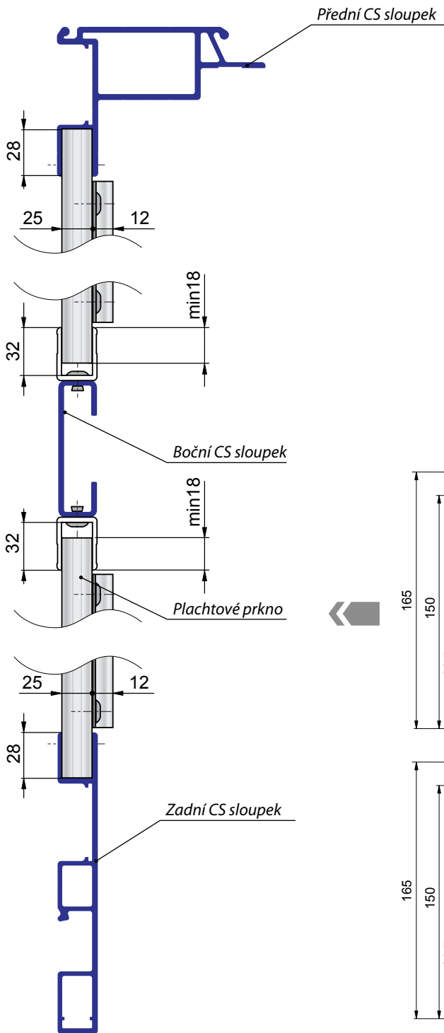
Obr. 4 Průřez nástavbou (horní pohled na řadu plachtových prken)
