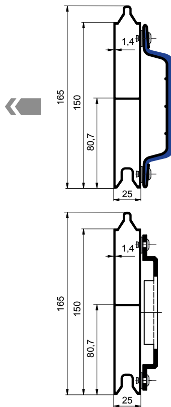
Obr. 3 Detail upevnění dvojitého plachtového prkna
