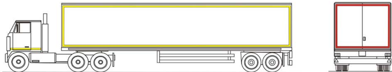
Obr. 5.: Bočné a zadné úplné odrazové označenie na návесе. Bočné úplné označenie môže byť použité namiesto predpísaného čiastočného označenia. Zadné úplné označenie zodpovedá predpísanej forme označenia. Na ťahači odrazové označenie nie je povinné, použitie líniového je len odporúčané.
