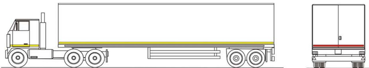
Obr. 3.: Bočné a zadné líniové odrazové označenie na návесе. Líniové označenie možno použiť iba vtedy, ak dodržanie predpísanej formy označenia nie je možné. Na ťahači odrazové označenie nie je povinné, použitie líniového je len odporúčané.
