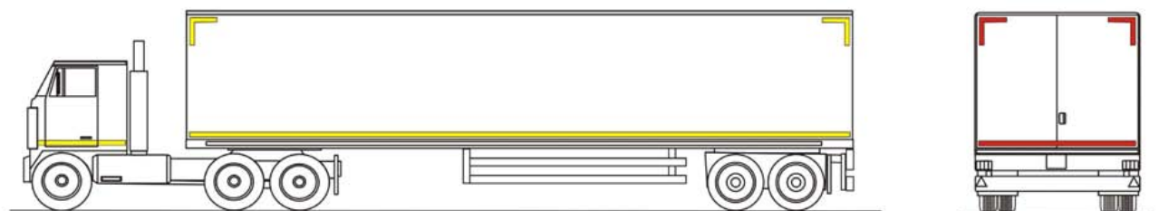
Obr. 4.: Bočné a zadné čiastočné odrazové označenie na návесе. Bočné čiastočné označenie zodpovedá predpísanej forme. Zadné čiastočné označenie možno použiť iba vtedy, ak dodržanie predpísanej formy označenia nie je možné. Na ťahači odrazové označenie nie je povinné, použitie líniového je len odporúčané.
