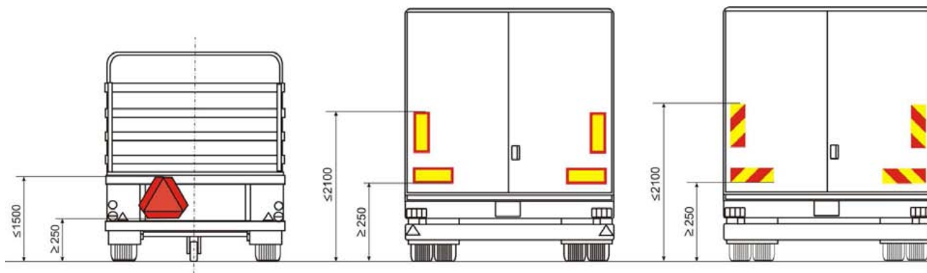
Obr. 1.: Dosiaľ povinné reflexné označenia vozidiel v SR. Vľavo označenie pomalého vozidla podľa predpisu EHK č. 69 (v SR do 40 km.h -1 ), uprostred označenie dlhého prípojného vozidla podľa predpisu EHK č. 70 (v SR vozidlá kategórií O1 až O3 dlhšie než 8 m vrátane oja a všetky vozidlá kategórie O4) a vpravo označenie ťažkého nákladného motorového vozidla podľa predpisu EHK č. 70 (v SR nad 7,5 t).
